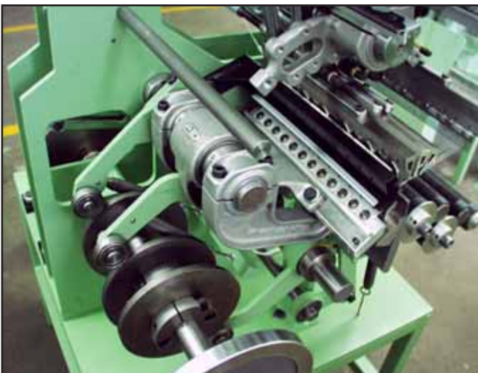
Antrieb der Wirkelemente über Kurvenscheiben drive to the knitting elements by cam discs
